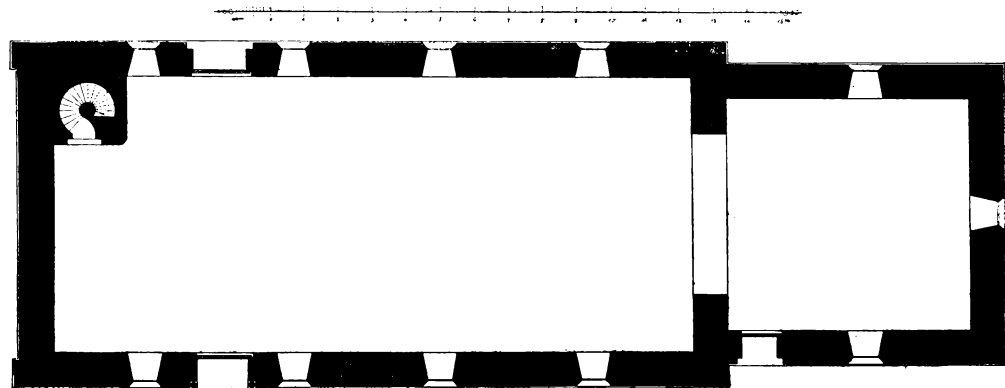
TAARNBORG KIRKE I SIN OPRINDELIGE SKIKKELSE. Tegnet af Arkitekt Erlangsen, Korsør.
